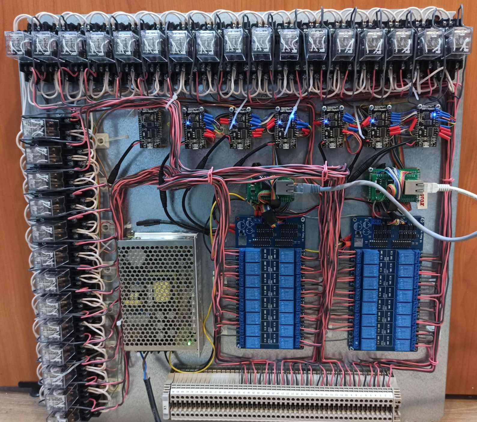
Модуль "Умный дом" на 30 нагрузок (Освещение, розетки, шлагбаум)
